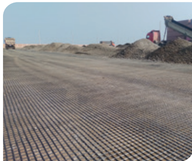
Refuerzo de base granular Puerto del Callao - Perú.
